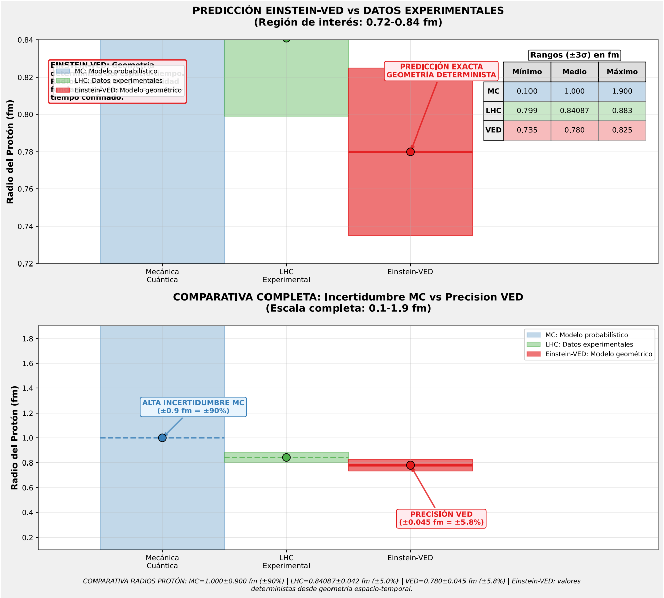
Figure 12 : Comparaison complète rayons protoniques - Échelle large montrant les différences
