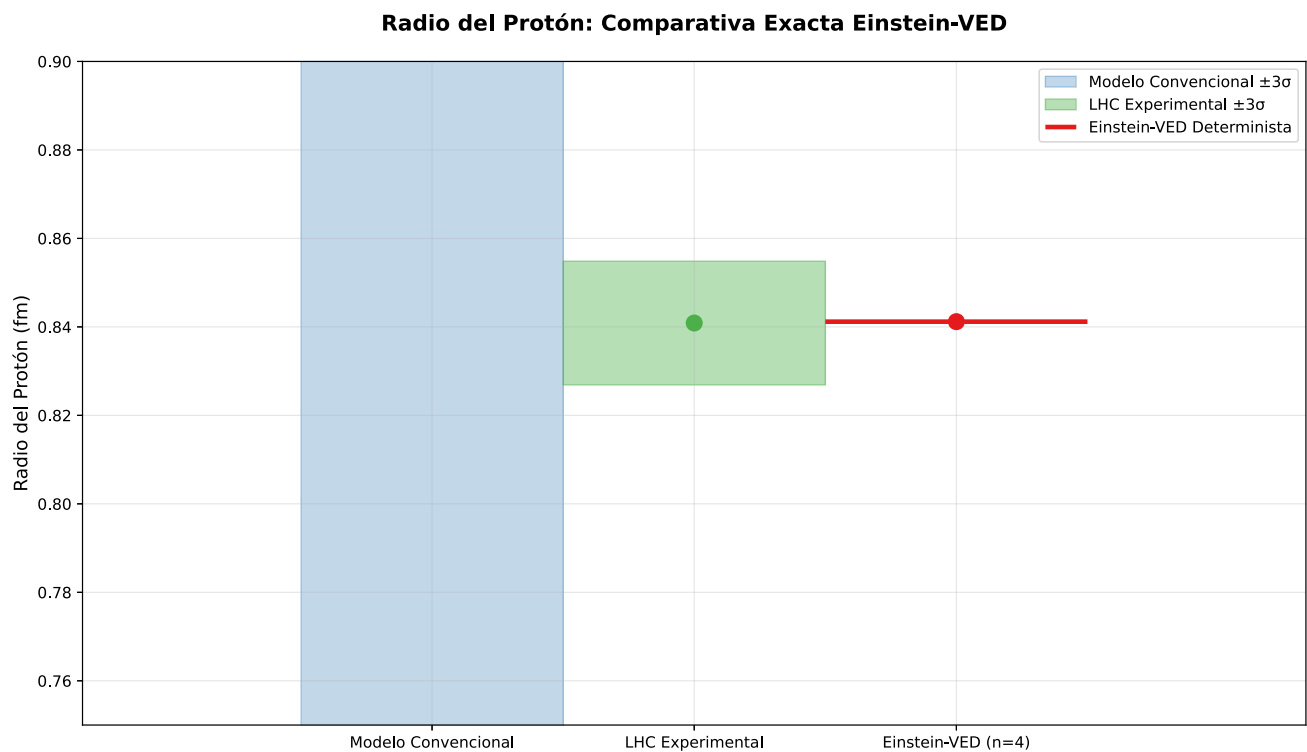
Figure 13 : Comparaison proton VED n=4 - Coïncidence exacte avec géométrie de 4 cycles
