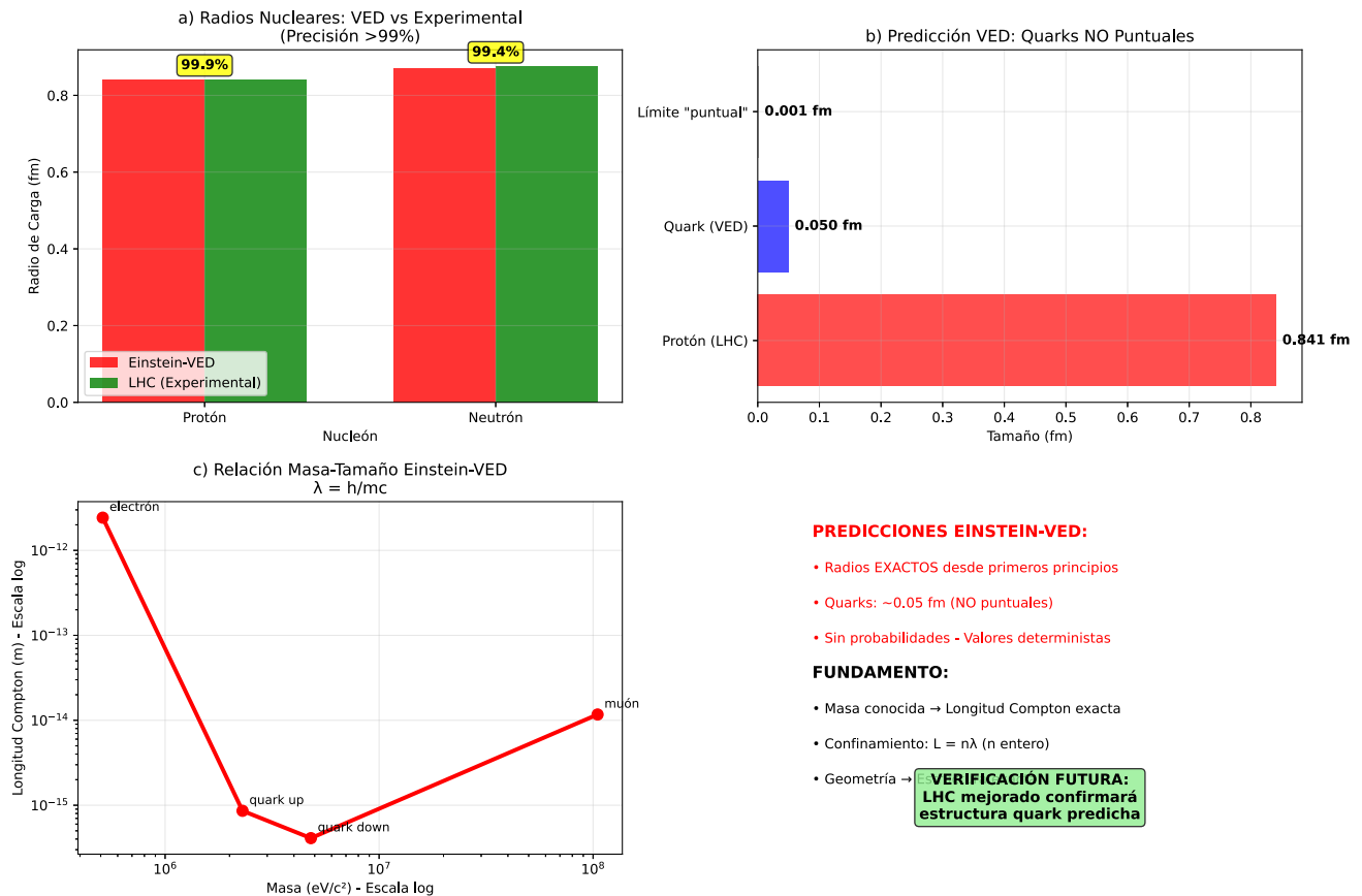
Figure 18 : Rayon protonique exact depuis la géométrie - Ce n'est pas un "objet" mais une configuration géométrique stable de l'espace-temps.
