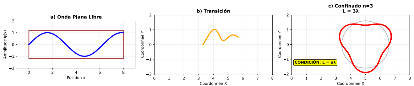
Figure 1 : Processus complet de confinement onde-particule - Transition d'une onde libre à une structure confinée stable
