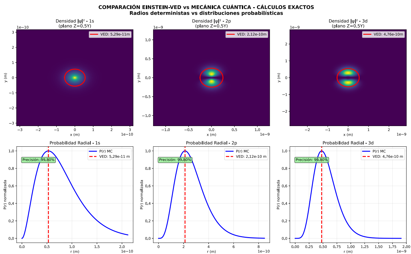
Figure 10 : Comparaison conceptuelle - Approche géométrique déterministe vs probabiliste
