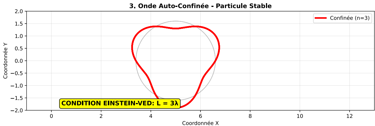
Figure 1d : État final - Onde auto-confinée stable avec résonance complète
