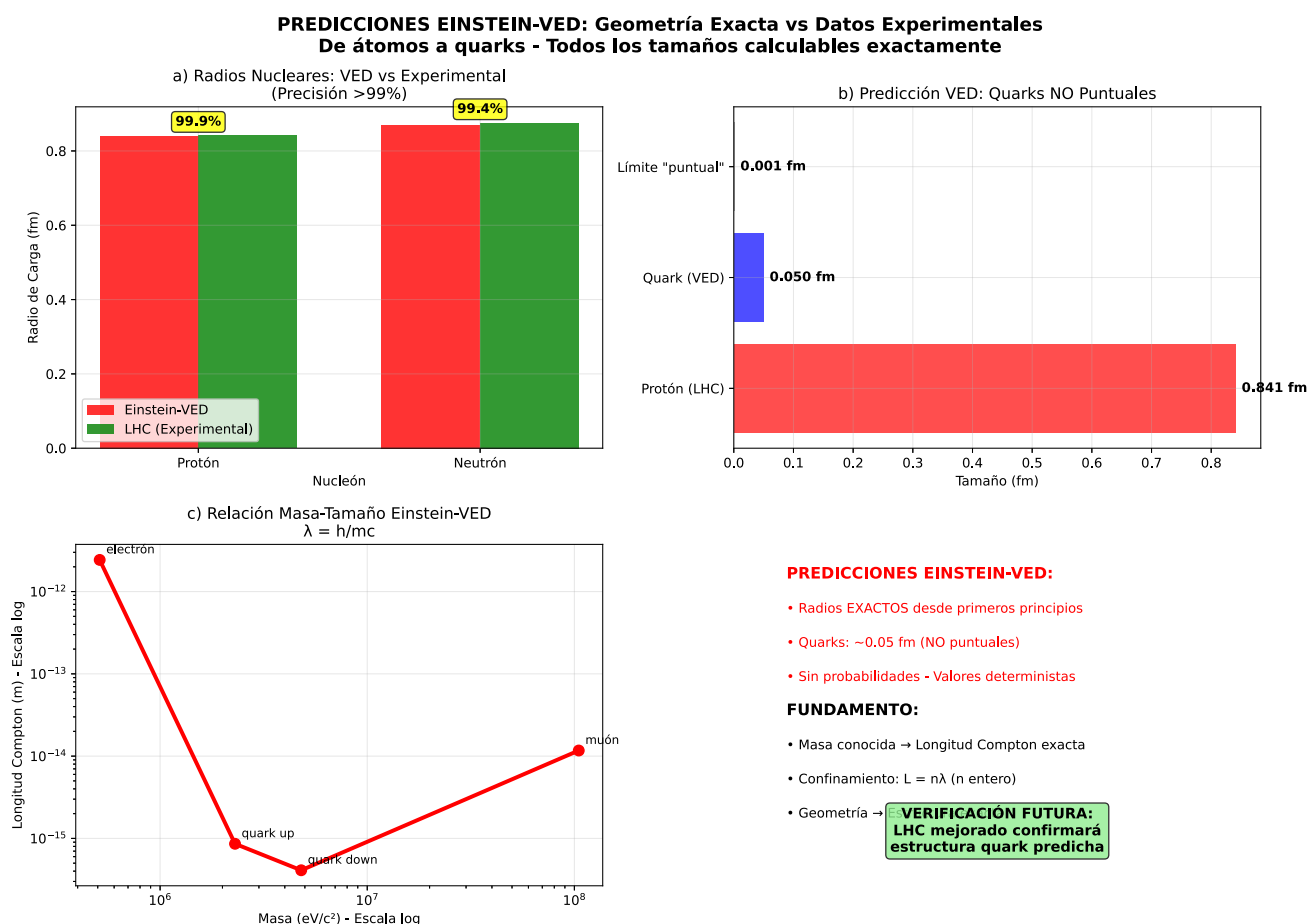
Figure 8 : Prédications Einstein-VED coïncident avec les données expérimentales du LHC avec précision >99% pour les rayons nucléaires
