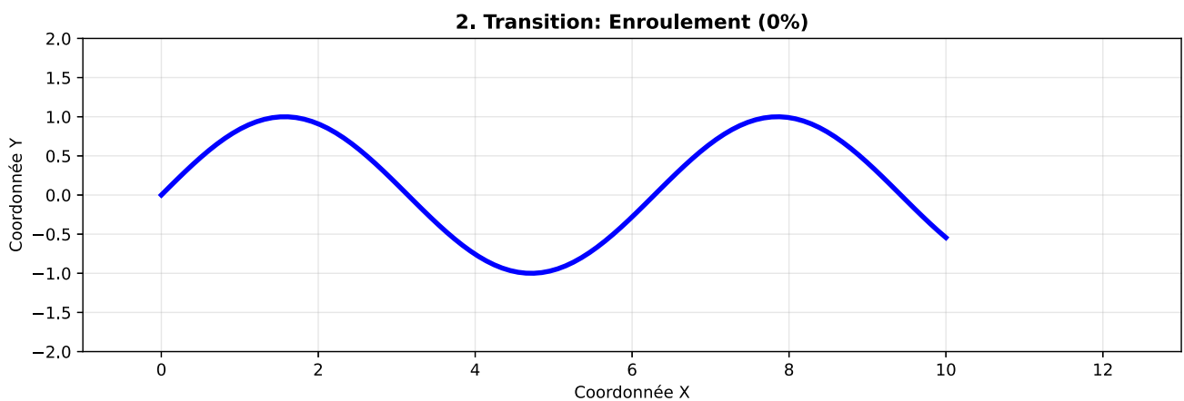
Figure 1b : Transition - Phase initiale d'enroulement progressif
