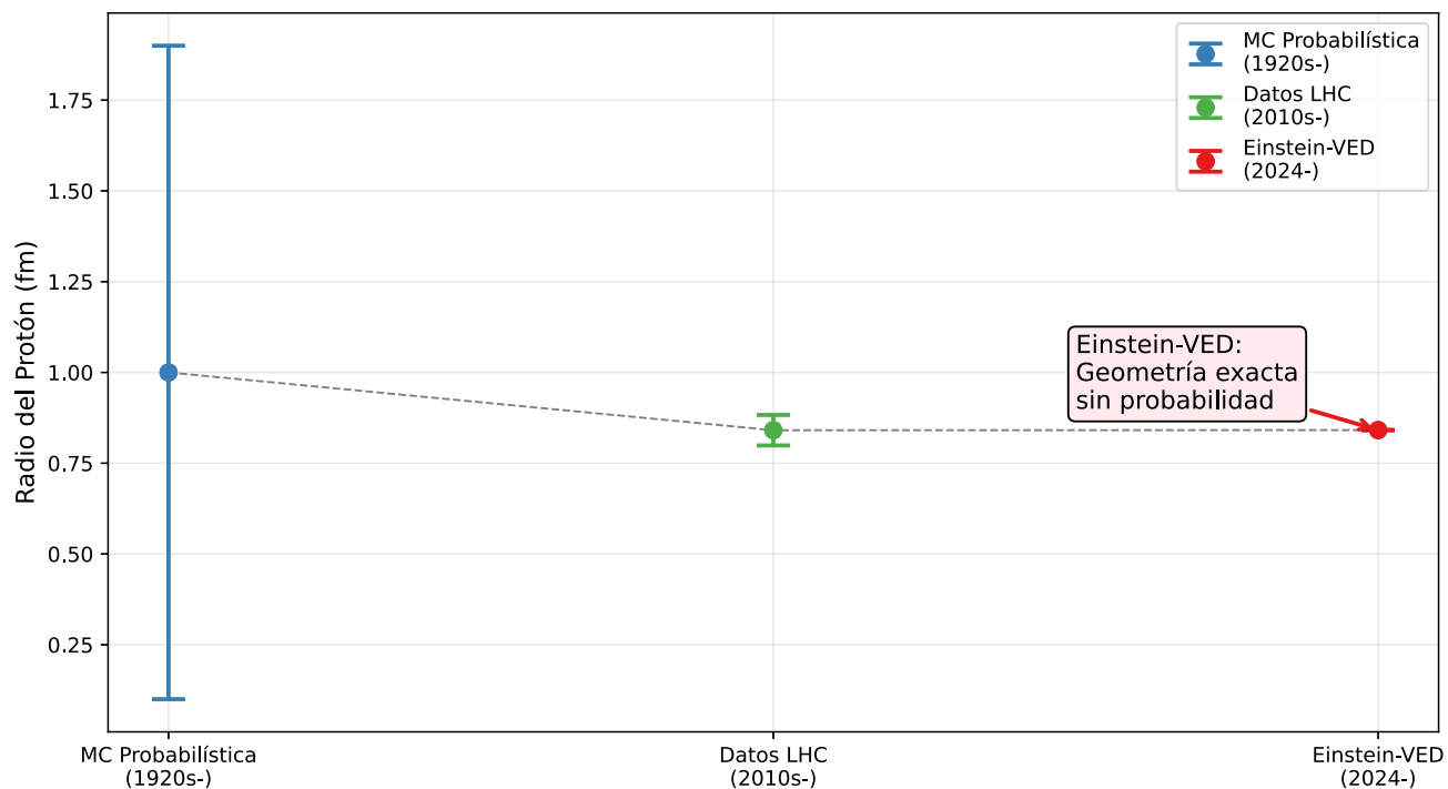
Figure 11 : Évolution théorique - De l'interprétation probabiliste à la géométrie déterministe
