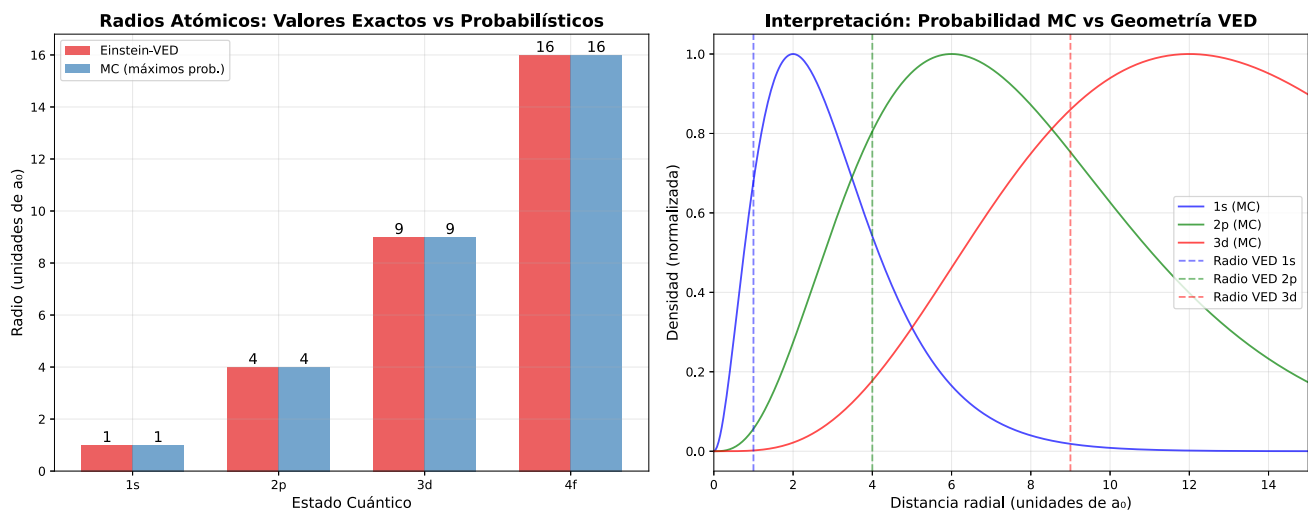
Figure 9 : Structures atomiques depuis la perspective Einstein-VED - Géométrie exacte vs interprétation probabiliste
